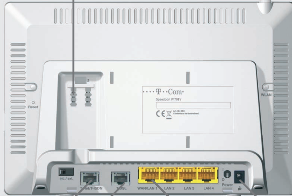
Speedport W 701V – Rückansicht mit Buchsenleiste
