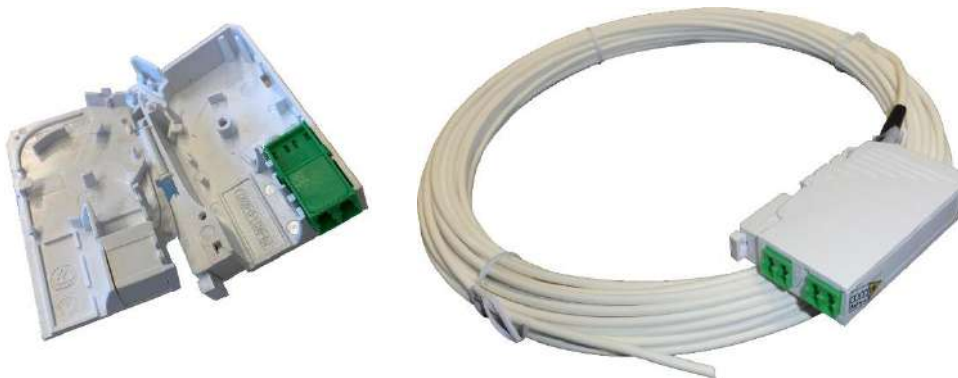
Abbildung 49: Gf-TA für ausschließliche Hutschiennenmontage (Quelle: Fa. Acome)
