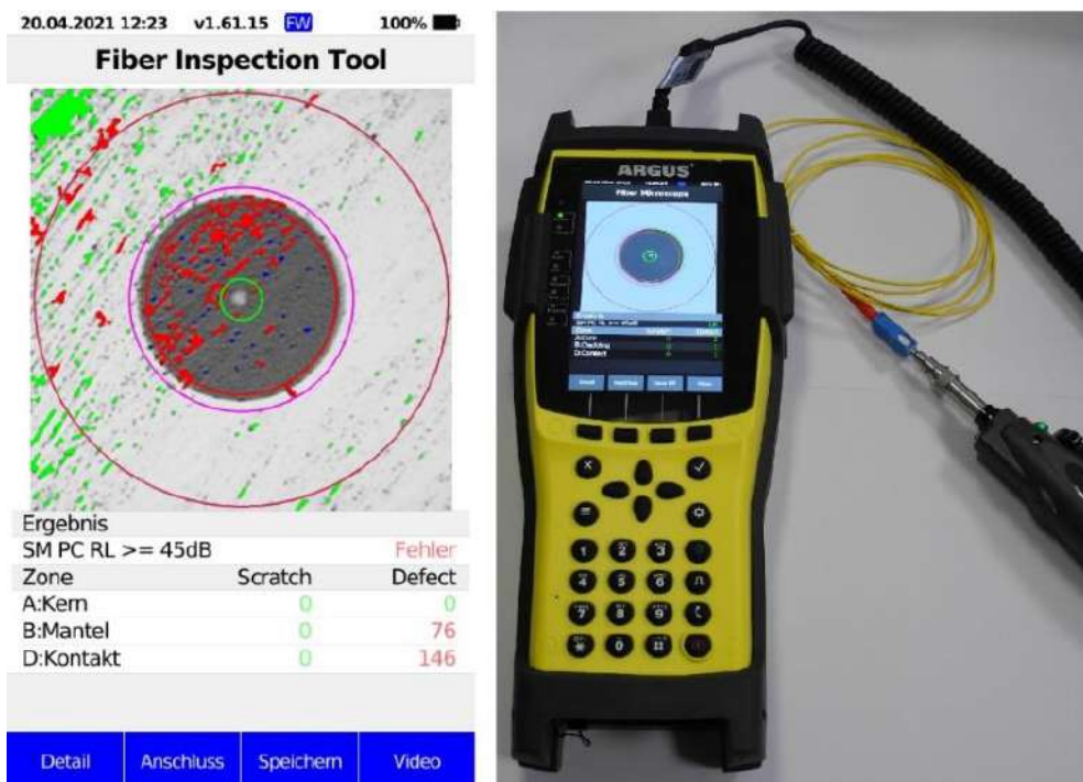
Abbildung 59: Fiber-Inspection-Tool (Quelle: Fa. intec)
