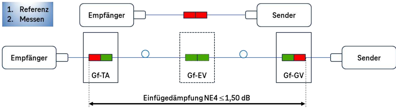
Abbildung 66: Messanschaltung Pegelmessgeräte – Normierung und Messung mit 2 Kabeln (Quelle: DT)
