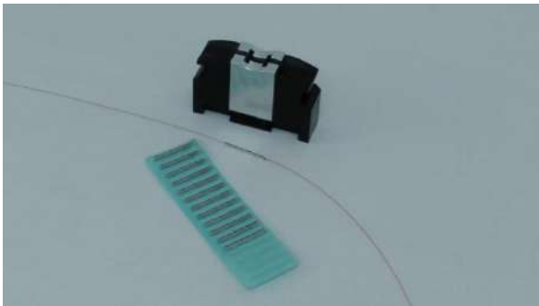
Abbildung 32: Krimpspleißschutz und zugehörige Presse (Quelle: Fa. Opternus)
