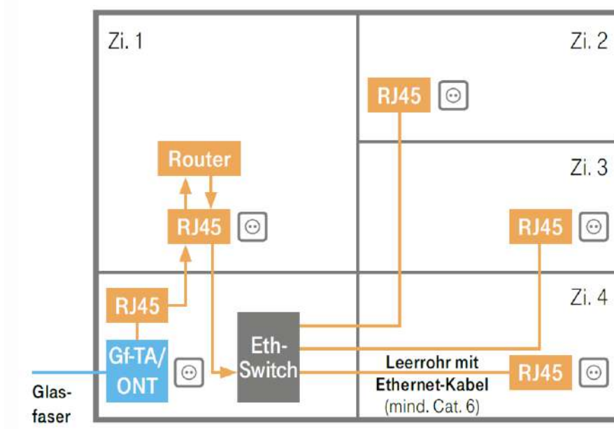
Abbildung 71: Prinzipdarstellung (Draufsicht) einer Verkabelung in einer Beispielswohnung (Quelle: DT)
