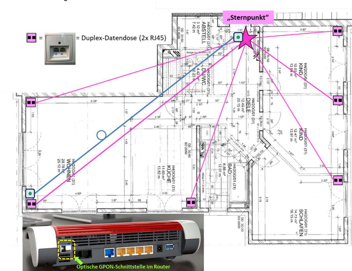
Abbildung 75: Einstieg in eine glasfaserbasierte Wohnungsverkabelung (Quelle: DT/AVM)
