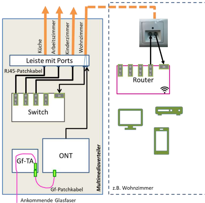
Abbildung 73: Prinzipdarstellung eines beschalteten Multimediaverteilers mit ausgelagertem Router (Quelle: DT)
