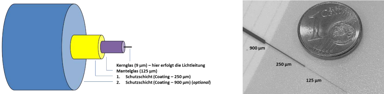
Abbildung 24: Schematischer Aufbau einer Glasfaser; 250 µm ↔ 900 µm (Quelle: DT)
