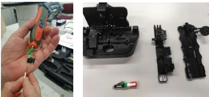
Abbildung 41: Herstellung LC-APC mit mech. Spleiß; li.: FO-Field, Fa. Reichle de Massari; re.: Fa. Corning (Quelle: DT)
