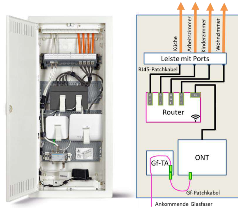
Abbildung 72: Beispiel eines beschalteten Multimediaverteilers (Quelle: links: Fa. Hager Electro; rechts: DT)
