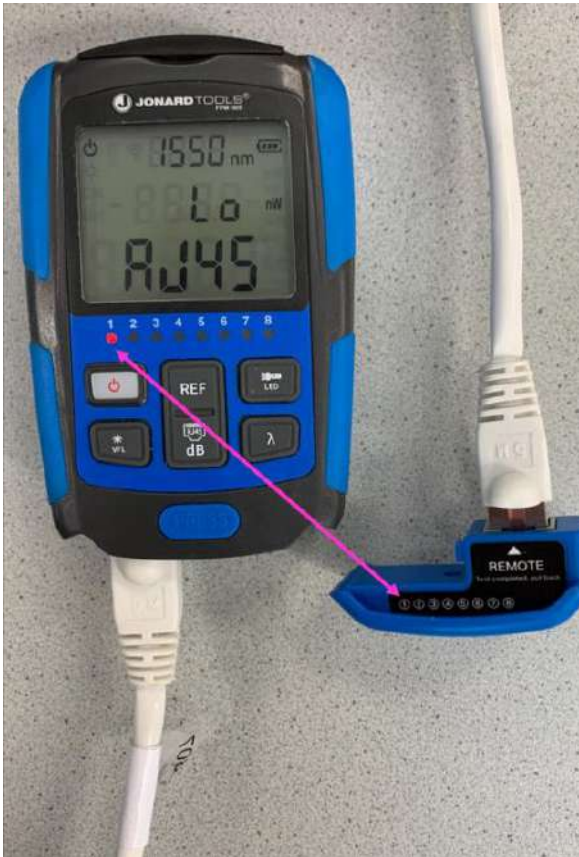
Abbildung 63: Optischer Pegelmesser FPM-50S als Kupfer-Netzwerkprüfgerät
