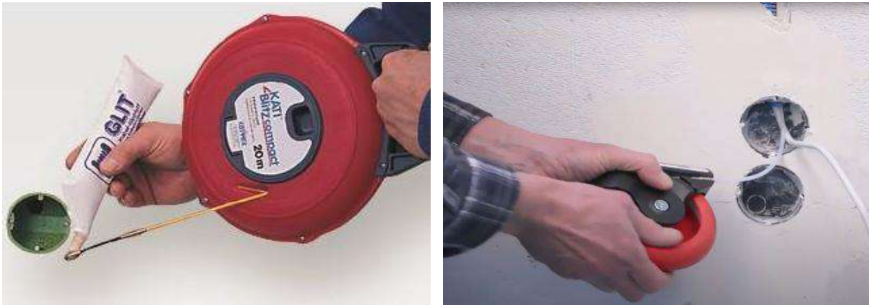
Abbildung 11: Auftragen von Kabelgleitmittel und Einziehgerät für belegte Leerrohre (Quelle: Fa. KATIMEX®)
