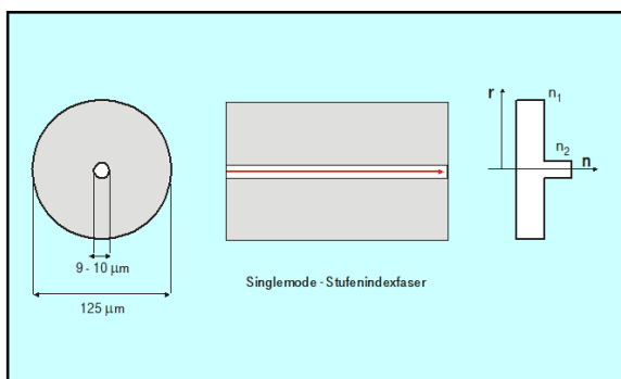
Abbildung 23: Singlemodefaser; Prinzipdarstellung Lichtleitung (Quelle: DT)
