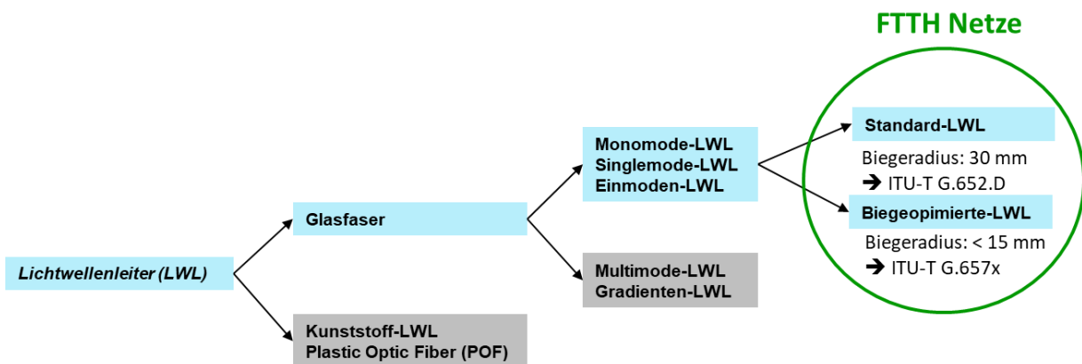
Abbildung 22: Übersicht und Einordnung verschiedener Lichtwellenleiter (Quelle; DT)
