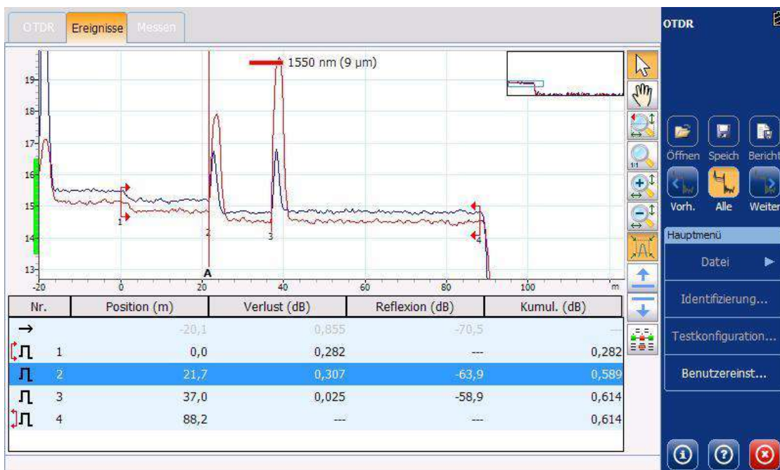
Abbildung 68: Typischen OTDR-Messkurve mit Zuordnung der gemessenen Ereignisse (Quelle: Fa. 3 Edge / Fa. EXFO)
