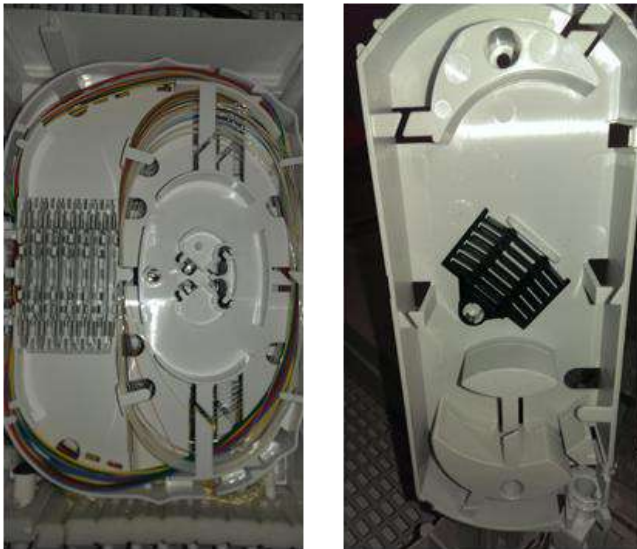
Abbildung 34: Beispielhafte Glasfaserspleißkassetten mit Spleißschutzaufnahmen (Quelle: DT)
