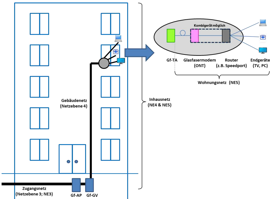
Abbildung 3: Netzebenen im Mehrfamiliengebäude (Quelle: DT)
