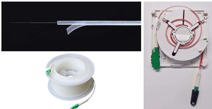
Abbildung 54: „Selbstklebendes transparentes Kabel“ in verschiedenen Produktvarianten (Foto: Fa. Huawei, DT)
