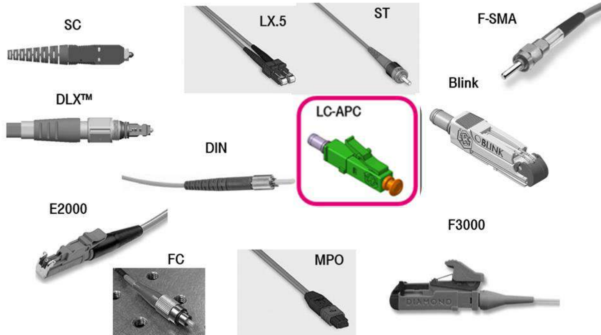
Abbildung 35: Auswahl an Glasfasersteckern (Quelle: DT)
