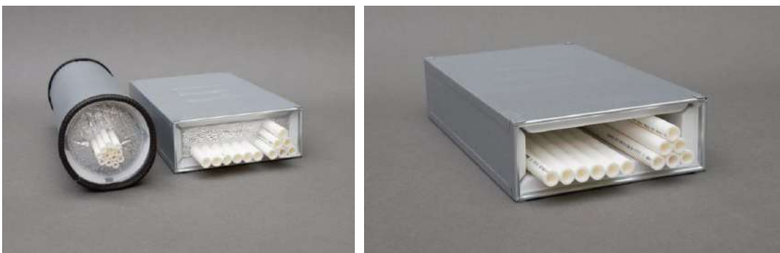
Abbildung 15: Wichmann Kabelbox (Quelle: Wichmann Brandschutzsysteme GmbH & Co. KG)
