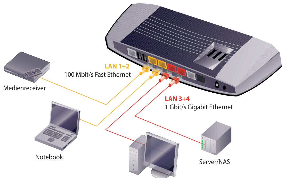
Abbildung 6 Computer anschließen
