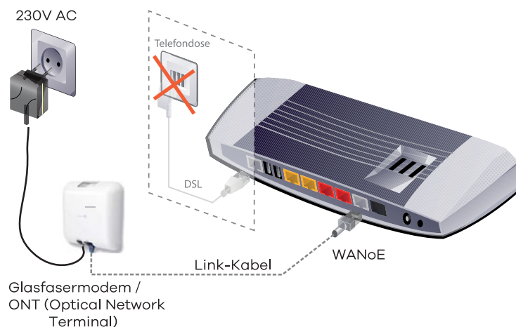
Abbildung 2 Anschlussvariante WAN over Ethernet
