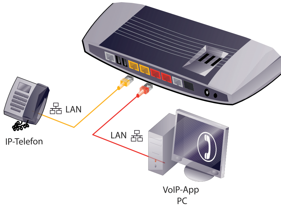
Abbildung 4 IP-Telefone anschließen
