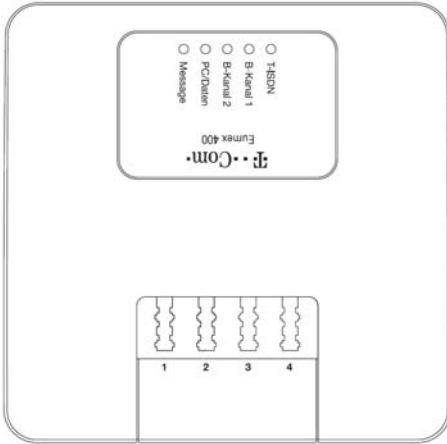
TAE-Buchsen und Leuchtdioden – Draufsicht von Eumex 400
