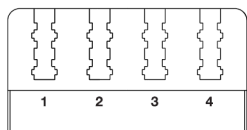
TAE-Buchsen von Eumex 400
