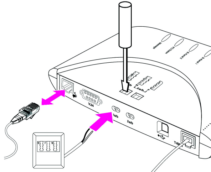
Anschluss einer abgesetzten TAE-Buchse, eines Telefons und eines Anrufbeantworters
