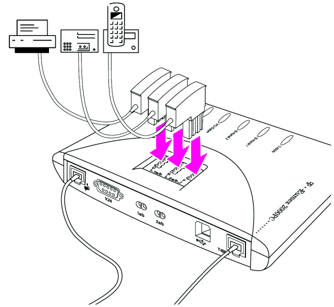
Anschluss eines Faxgerätes, eines Telefons und eines Anrufbeantworters
