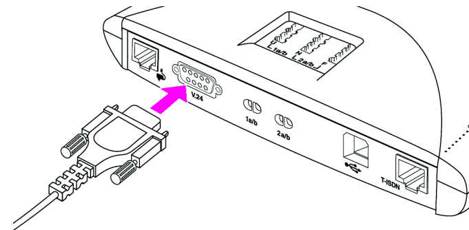
Anschluss des Computers über die V.24-Schnittstelle von T-Eumex 2000PC
