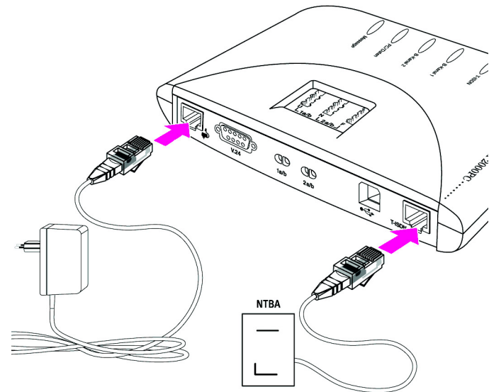
Anschluss von T-Eumex 2000PC an das ISDN und die Stromversorgung
