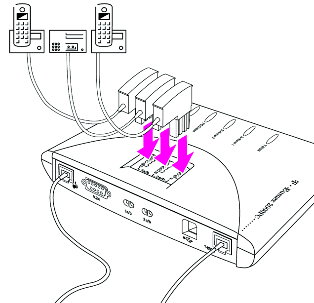
Anschluss von zwei Telefonen und einem Anrufbeantworter
