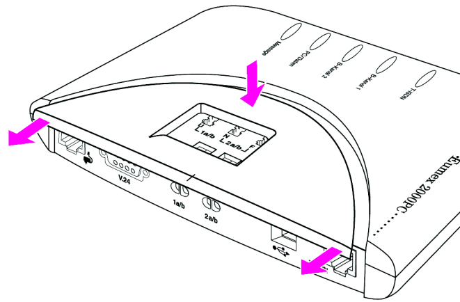
Entfernen der Abdeckung von T-Eumex 2000PC
